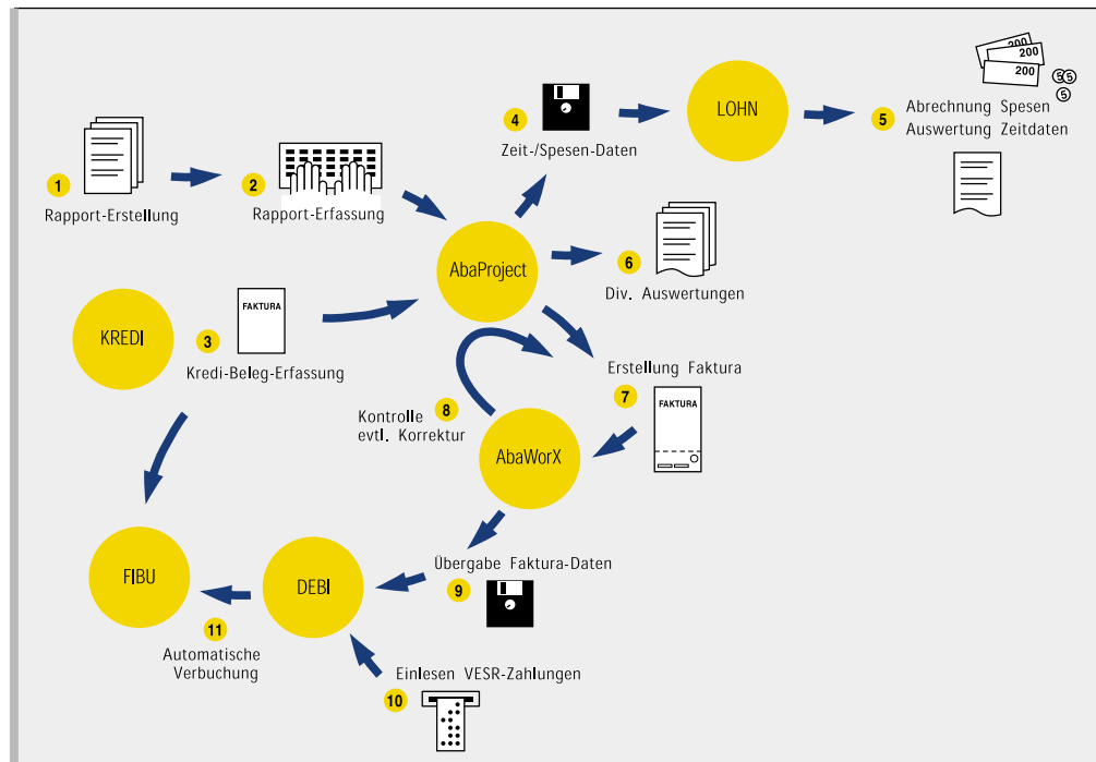
ABACUS Gesamtlösung mit AbaProject: Datenfluss
